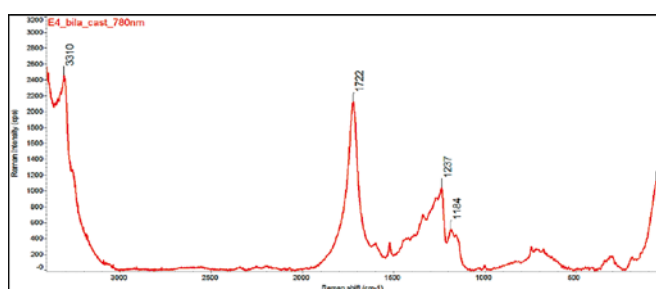
Graf 5: Ramanovo spektrum 780 nm, vzorek E4 – bílá část (autor analýzy P. Antoš).
